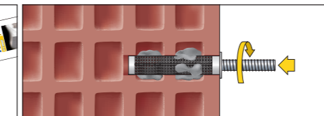
5. Ankerstange drehend eindrücken
