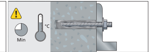
5. Vor der Montage und Aufbringen eines Drehmoments Aushärtezeit beachten
