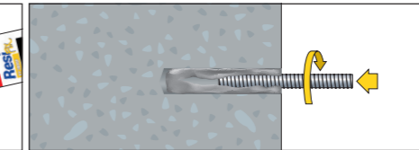
4. Ankerstange drehend eindrücken
