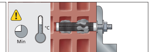
6. Vor der Montage und Aufbringen eines Drehmoments Aushärtezeit beachten
